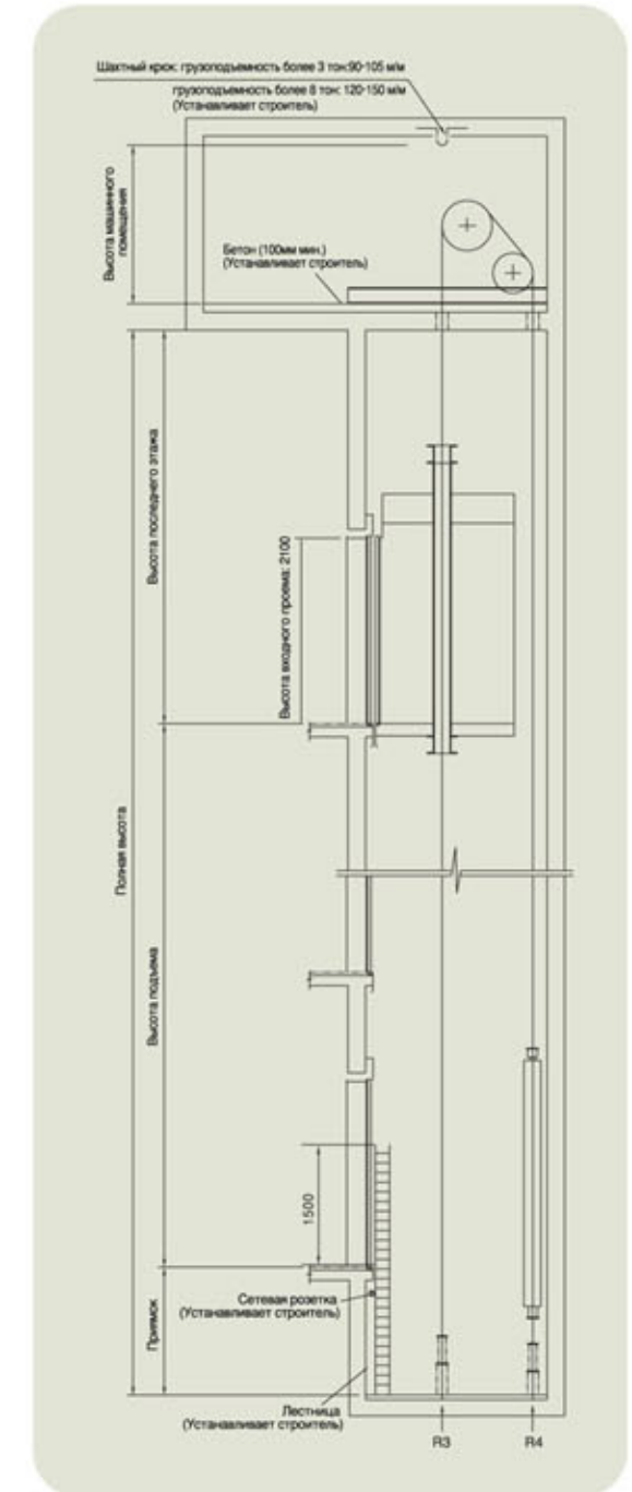
СЕЧЕНИЕ ШАХТЫ
