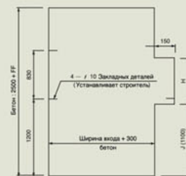
Строительный план здания
