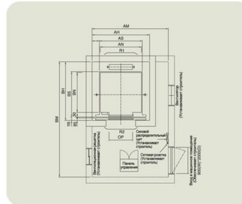
ПЛАН ШАХТЫ И МАШИНОГО ПОМЕЩЕНИЯ (система контроля- одиночное управление)
