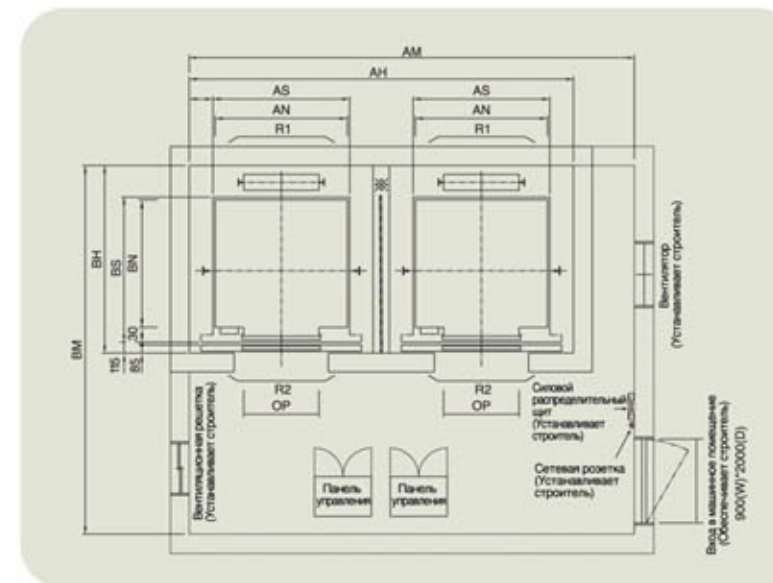
ПЛАН ШАХТЫ И МАШИНОГО ПОМЕЩЕНИЯ (система контроля- парное управление)
